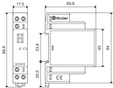
Type 22.34 Bornes à cage
