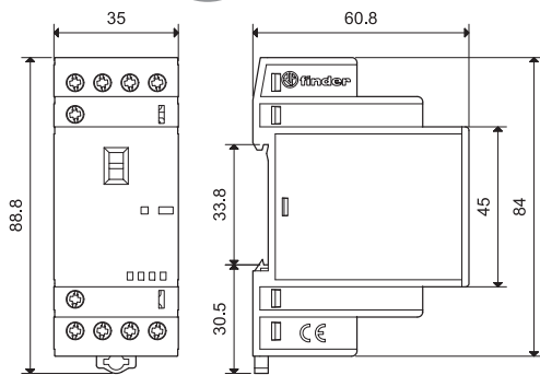
Type 22.44 / 22.64 Bornes à cage
