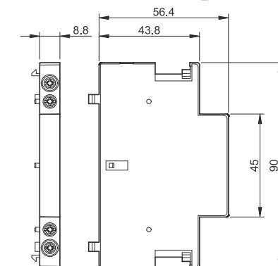
Type 022.63 / 022.65 Bornes à cage
