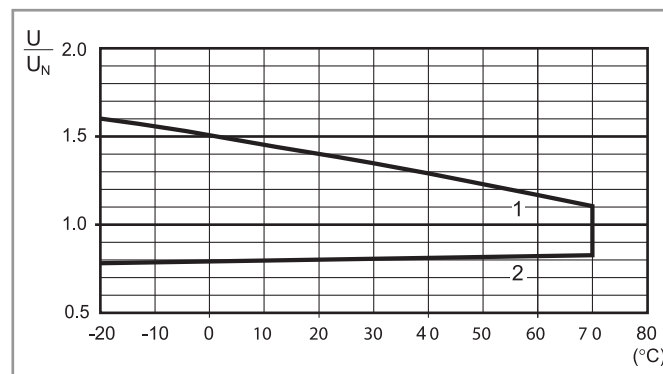
R 60 - Plage de fonctionnement bobine AC en fonction de la température ambiante
