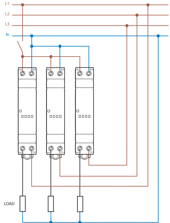
Exemple de connexion en triphasé (avec 3 x 77.01.8.230.8051)
