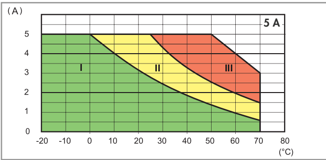
L77-1 Courant efficace maximum en fonction de la température ambiante 77.01.0.024.805x @ 32 V DC
