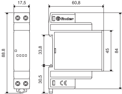
77.x5 Bornes à vis
