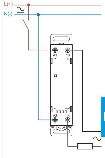
Connexion en monophasé (77.31.....7x)
