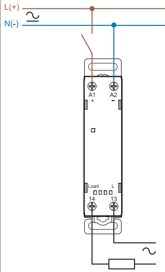
Connexion en monophasé (77.11)
