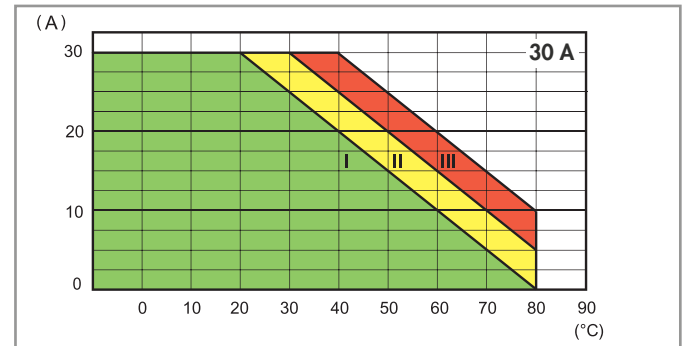
L77-4 Courant efficace maximum en fonction de la température ambiante 77.31.x.xxx.80xx
