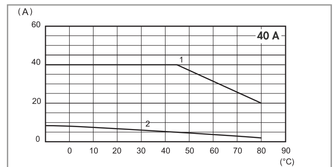
L77-9 Courant efficace maximum en fonction de la température ambiante 77.45.x.xxx.8x50
