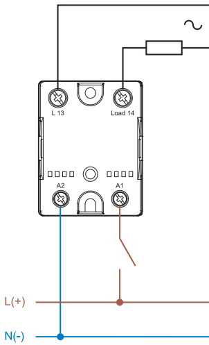
Connexion en monophasé (77.x5)
